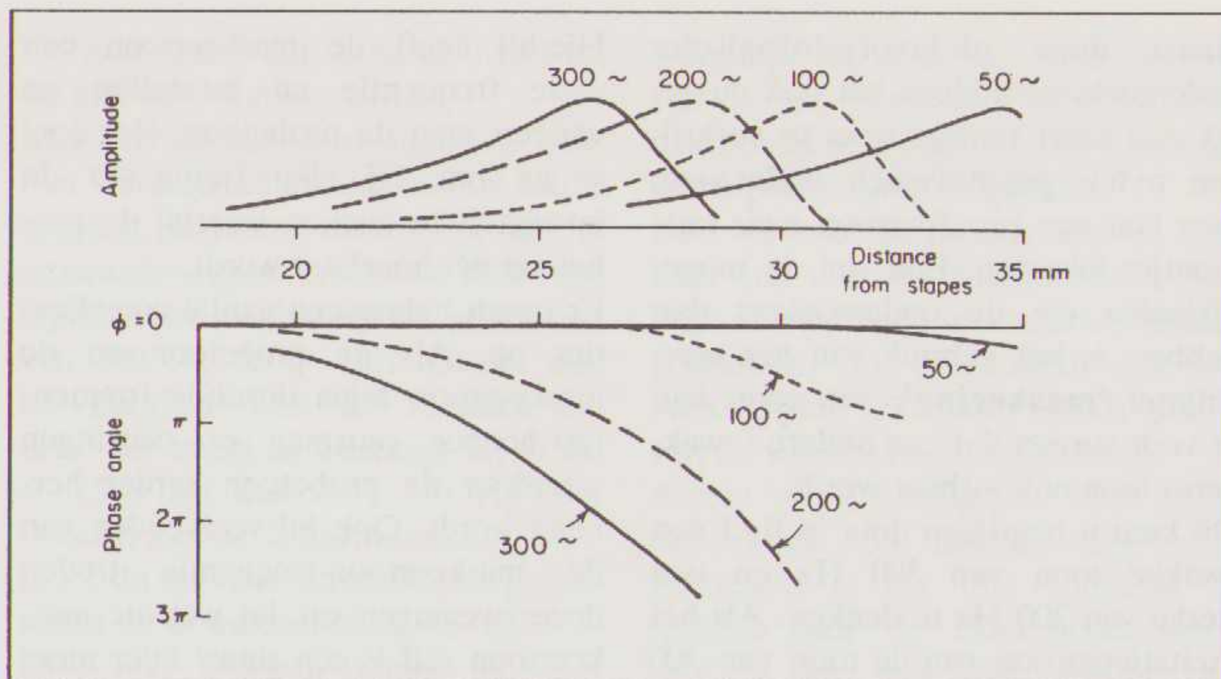
Figuur 1. Excitatiepatronen (omhullenden) van het basilair membraan voor verschillende stimulusfrequenties (naar v. Bekesy,
